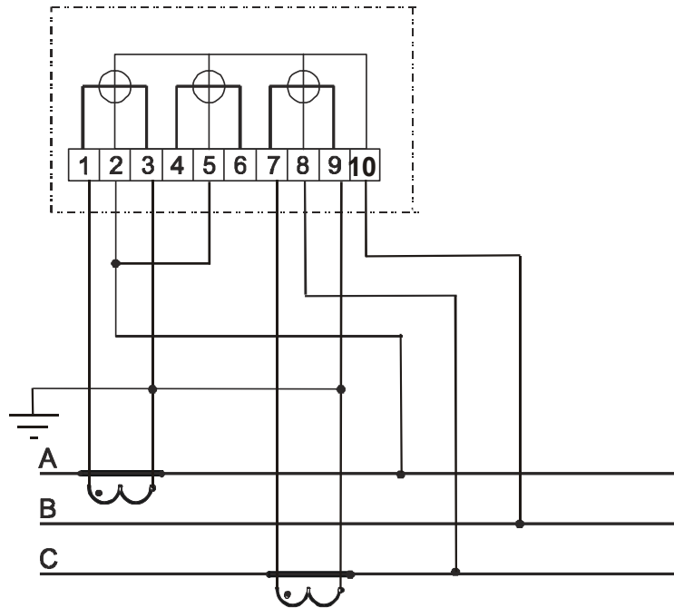
Рисунок Б.9 - Схема включения трехэлементного счетчика в трехпроводную сеть напряжением 0,22 кВ с изолированной нейтралью
