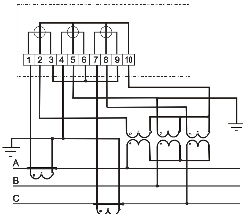
Рисунок Б.8 - Схема включения трехэлементного счетчика в трехпроводную сеть с тремя трансформаторами напряжения и заземленной фазой В
