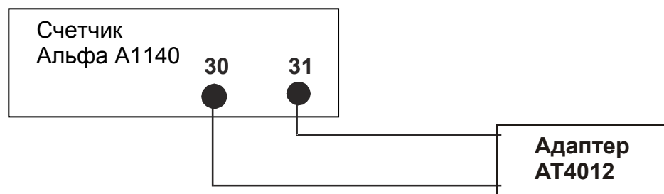
Рисунок Б.11 – Подключение к счетчику Альфа А1140 адаптера резервного питания
