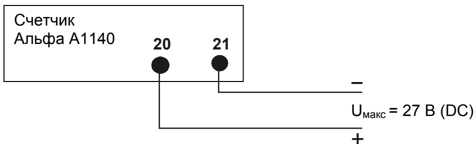
Рисунок Б.10 – Подключение импульсного выхода счетчика Альфа А1140 (при отсутствии дополнительного питания)
