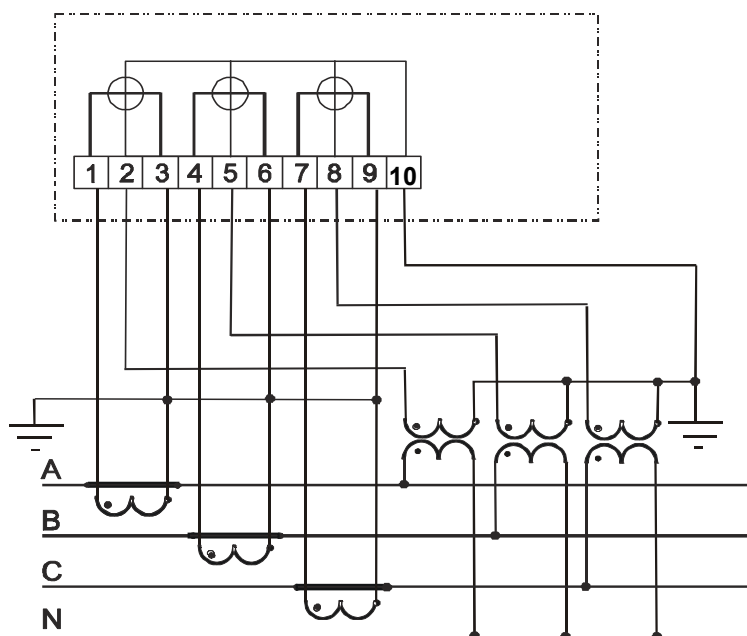
Рисунок Б.4 - Схема включения трехэлементного счетчика в четырехпроводную сеть с заземленной нейтралью
