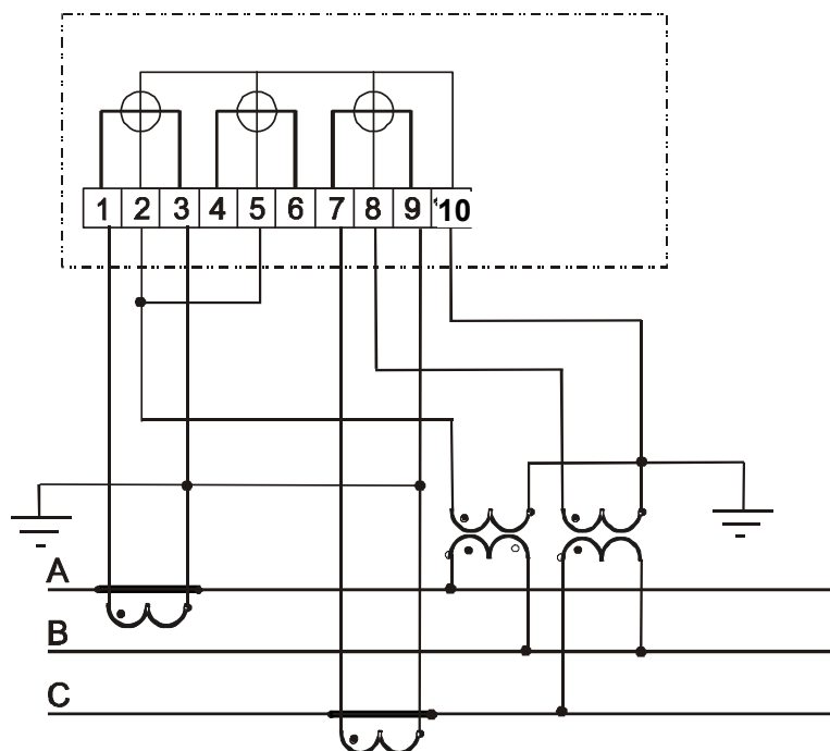
Рисунок Б.6 - Схема включения трехэлементного счетчика в трехпроводную сеть с двумя трансформаторами напряжения
