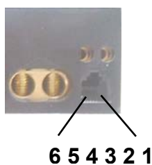
Рисунок 4 - Расположение контактов разъема RJ12 счетчика
