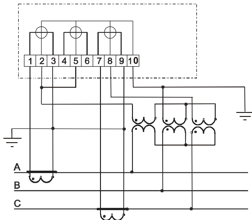
Рисунок Б.7 - Схема включения трехэлементного счетчика в трехпроводную сеть с тремя трансформаторами напряжения и заземленной фазой В
