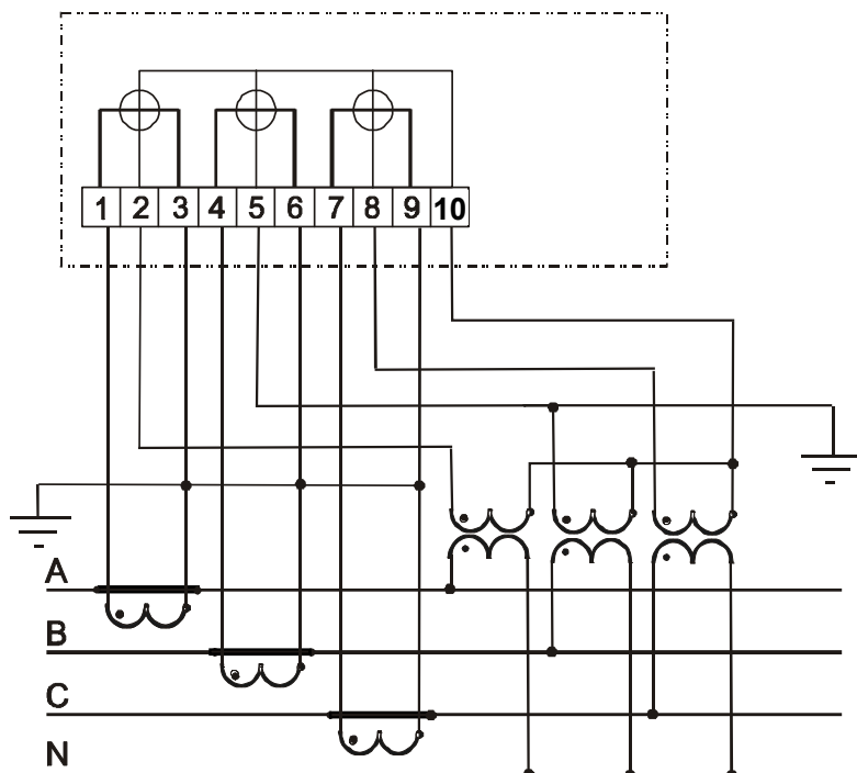
Рисунок Б.5 - Схема включения трехэлементного счетчика в четырехпроводную сеть с изолированной нейтралью и заземленной фазой В
