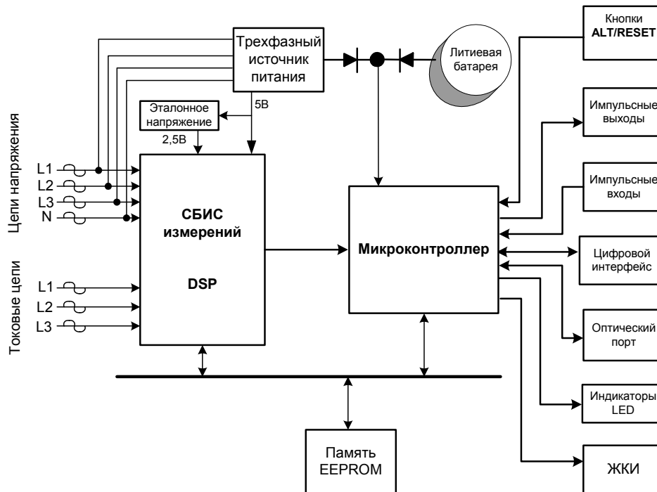
Рисунок 2 – Структурная схема счетчика Альфа А1140
