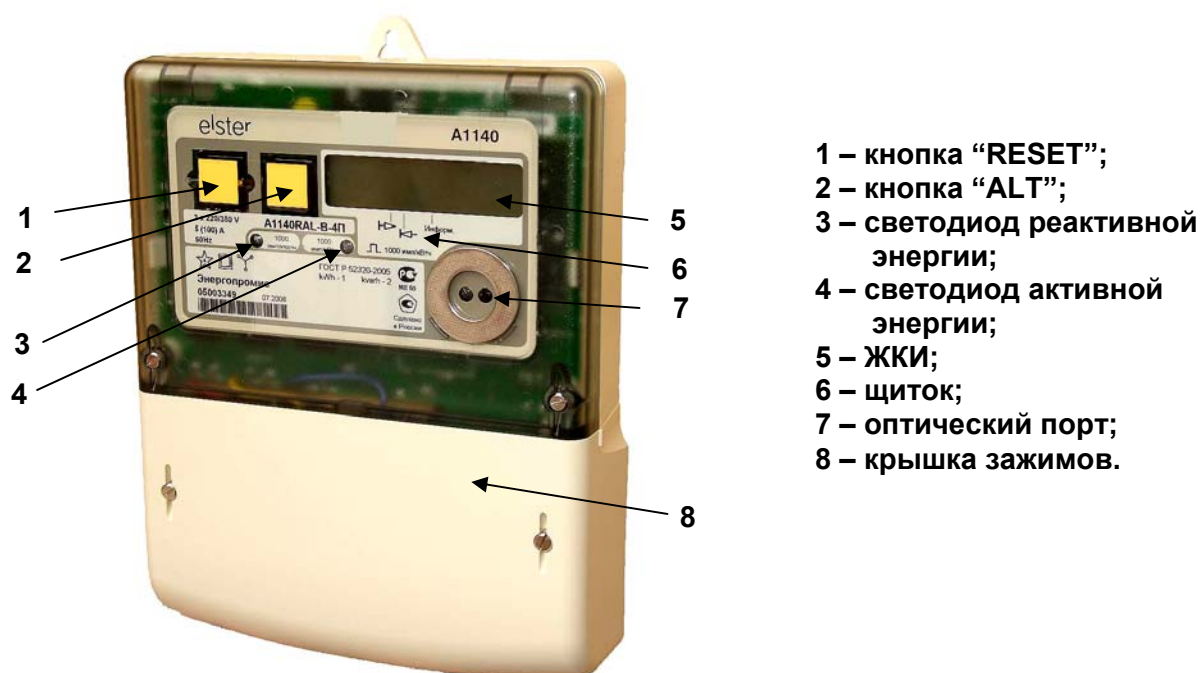
Рисунок 1 - Внешний вид счетчика Альфа А1140
