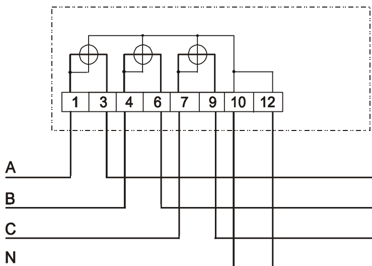
Рисунок Б.1 - Схема подключения счетчика прямого включения в четырехпроводную сеть напряжением 0,4 кВ
